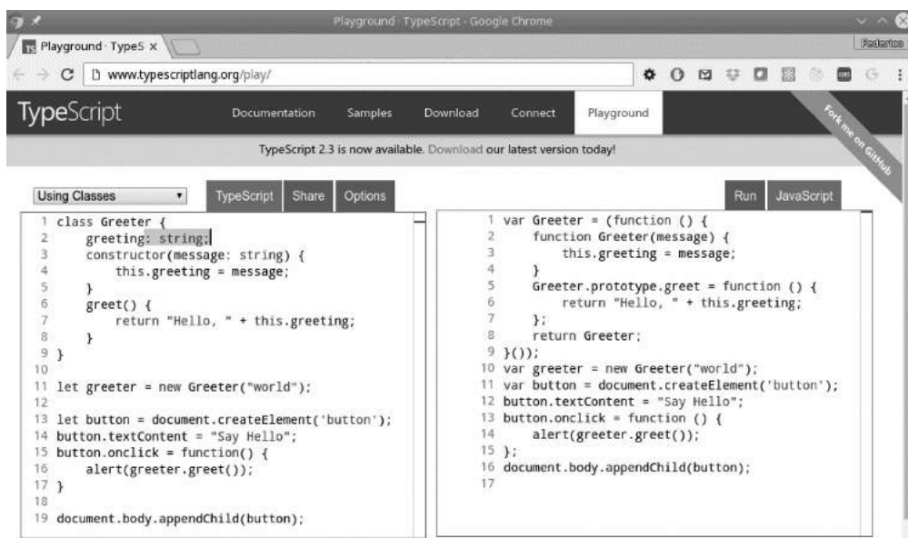
Slika 1.4 TypeScript dodaje funkcije provere tipa za bezbednije programiranje.
