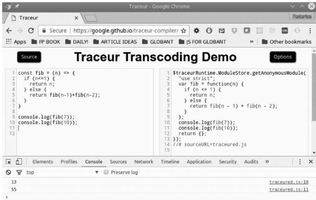
Slika 1.3 Transpajler Traceur podjednako je validna alternativa za prevod ES10 koda u JS5 kod.
